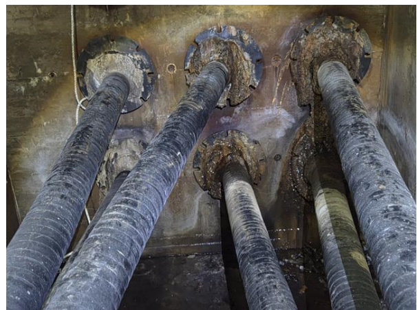
내용 종점벽체 Sta.32m 관로구 누수
